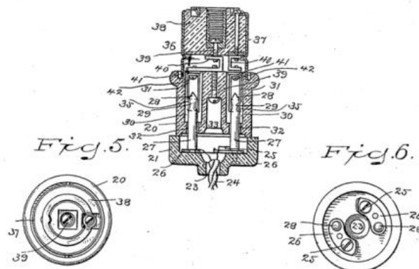
Tekening van eerste elektrische stopcontact (VS-patent: 774,250)
